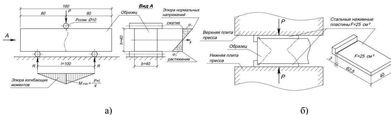
Рис. 10. Схема испытания а) изгиб б) сжатие
