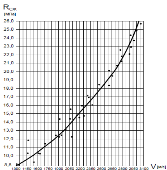
Рис. 13. Градуировочная зависимость «скорость–прочность»
