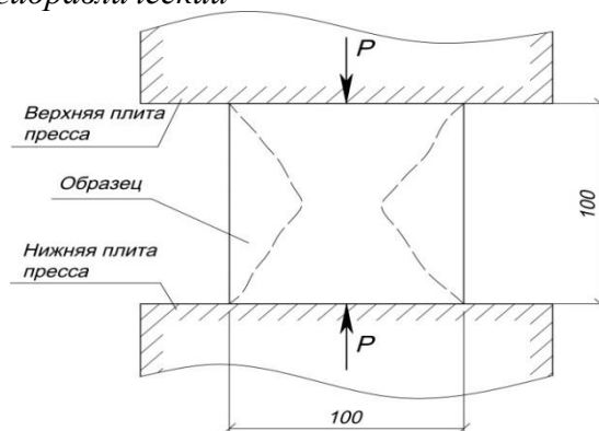
Рис. 17. Схема испытания
