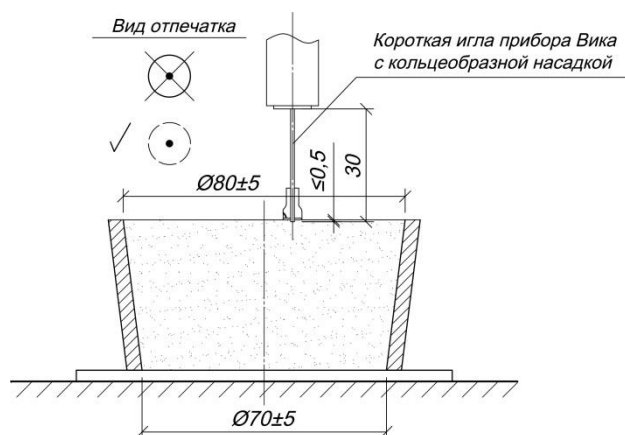
Рис. 5. Схема определения конца схватывания
