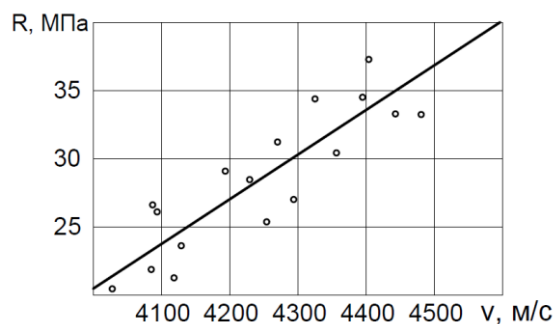
Рис. 15. Градуировочная зависимость «скорость–прочность»
