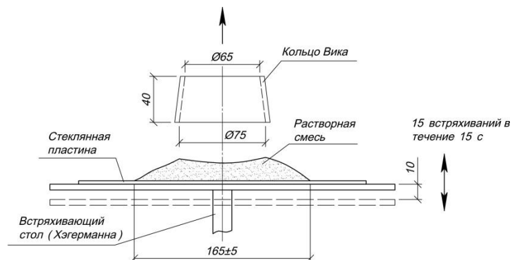
Рис. 13. Схема испытания
