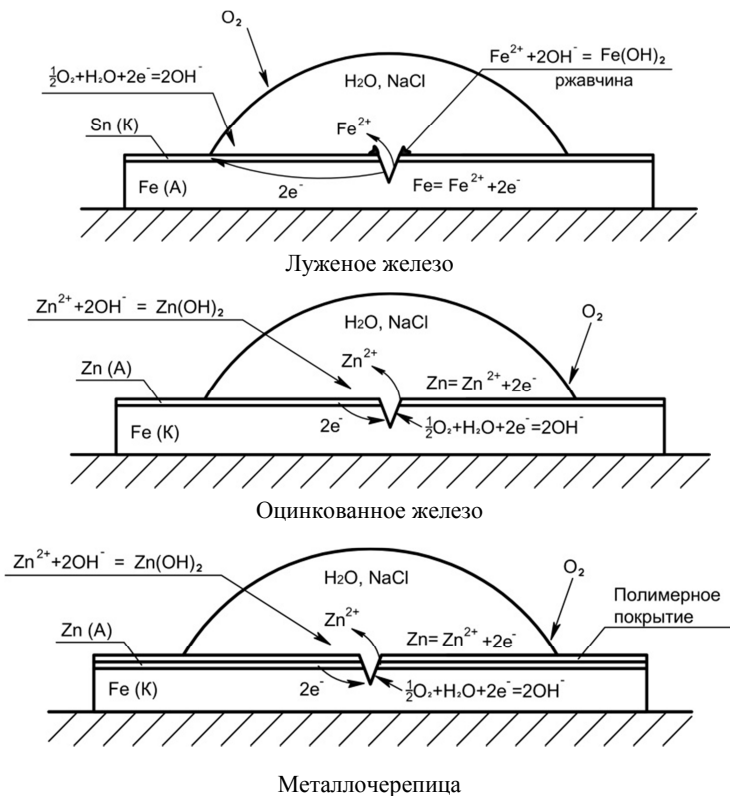
Рис. 5. Схемы коррозионных процессов
