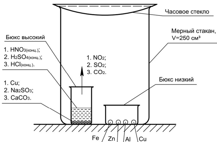
Рис. 1. Схема испытания
