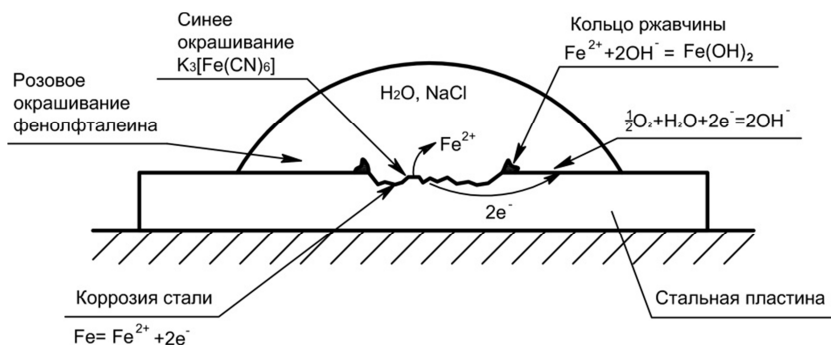
Рис. 4. Схема коррозии стали при неравномерной аэрации
