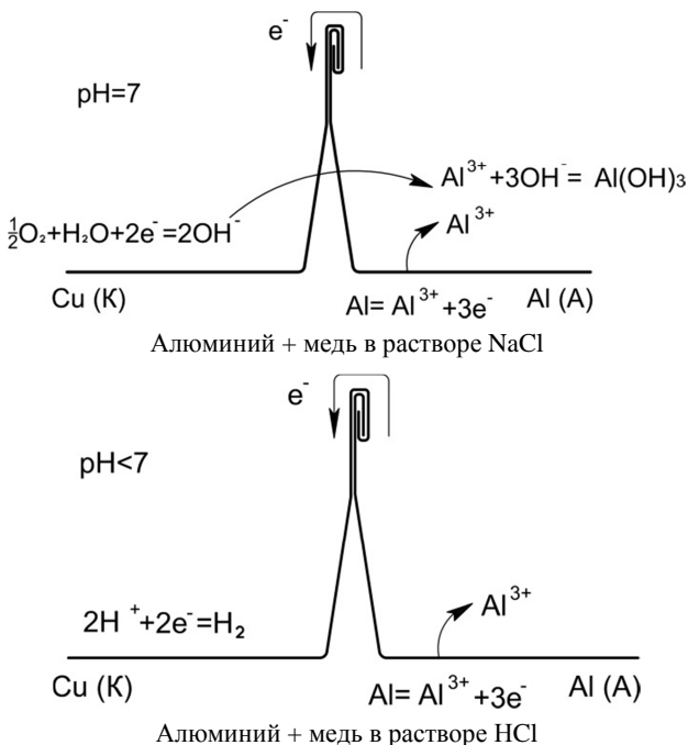
Рис. 3. Схемы образовавшихся коррозионных гальванических элементов
