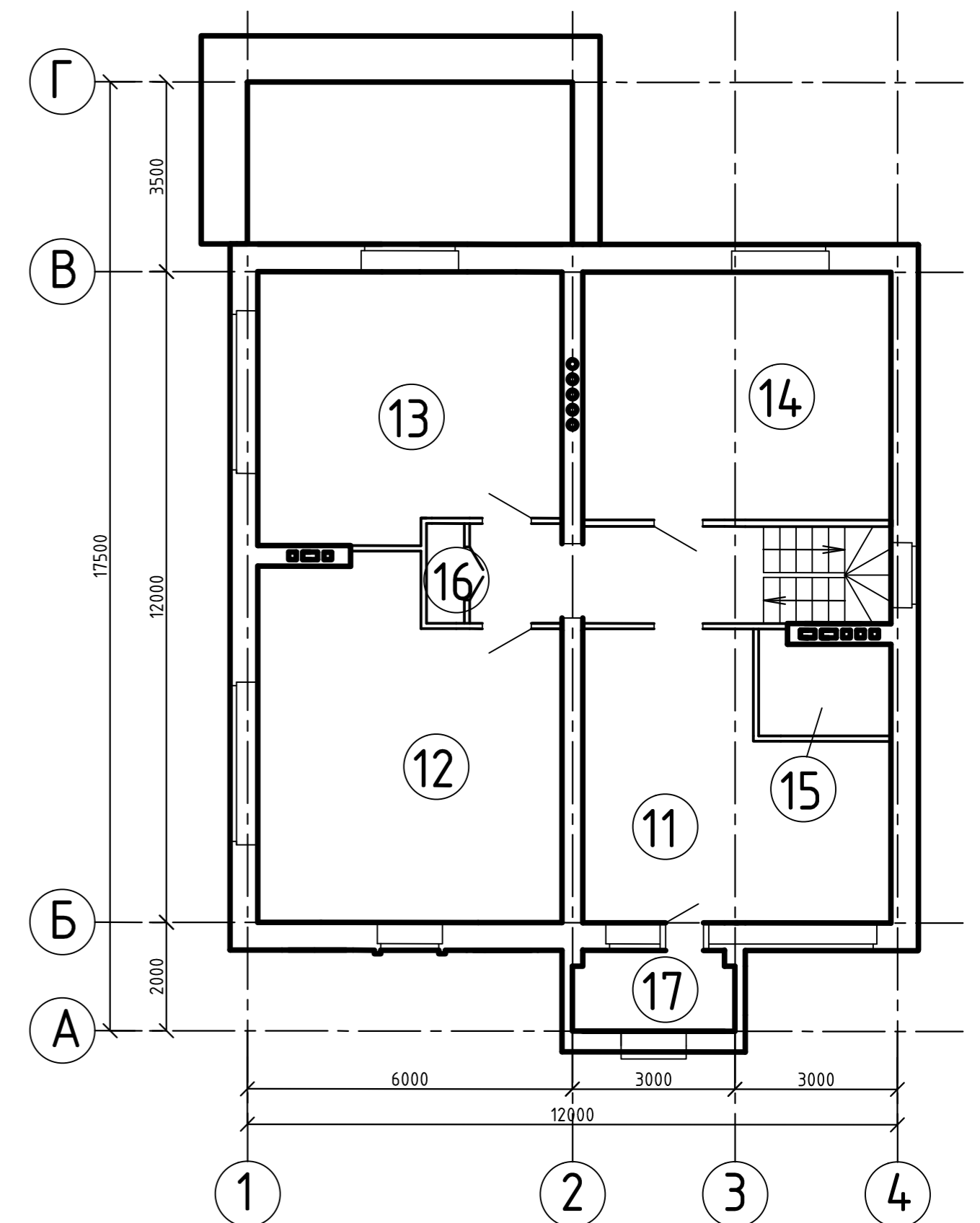
ПЛАН ВТОРОГО ЭТАЖА М 1:100
