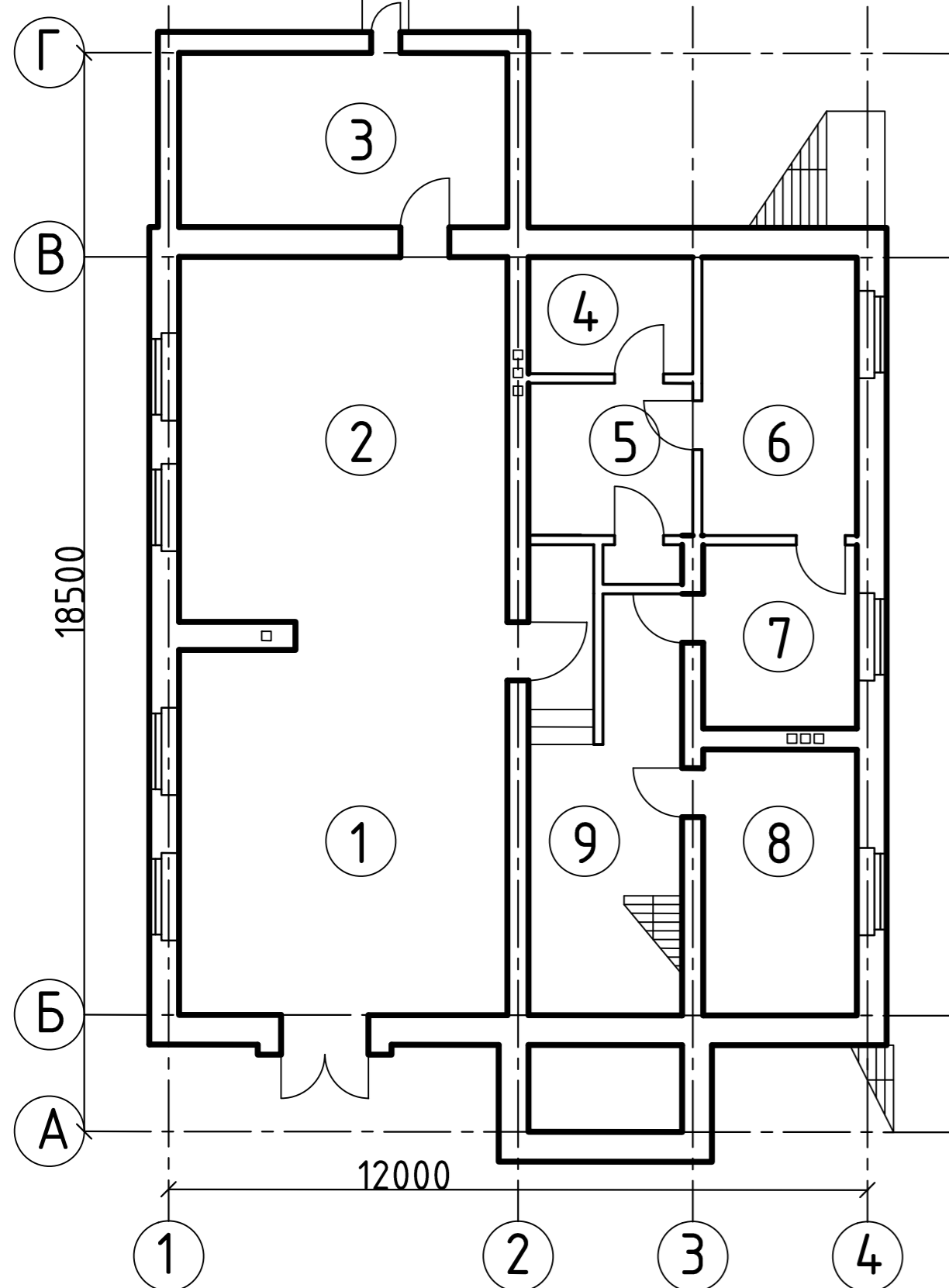
ПЛАН ЦОКОЛЬНОГО ЭТАЖА М 1:100
