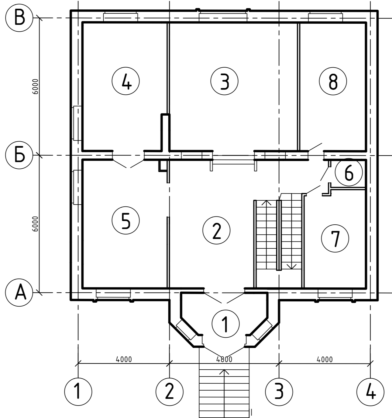
ПЛАН ПЕРВОГО ЭТАЖА М 1:100
