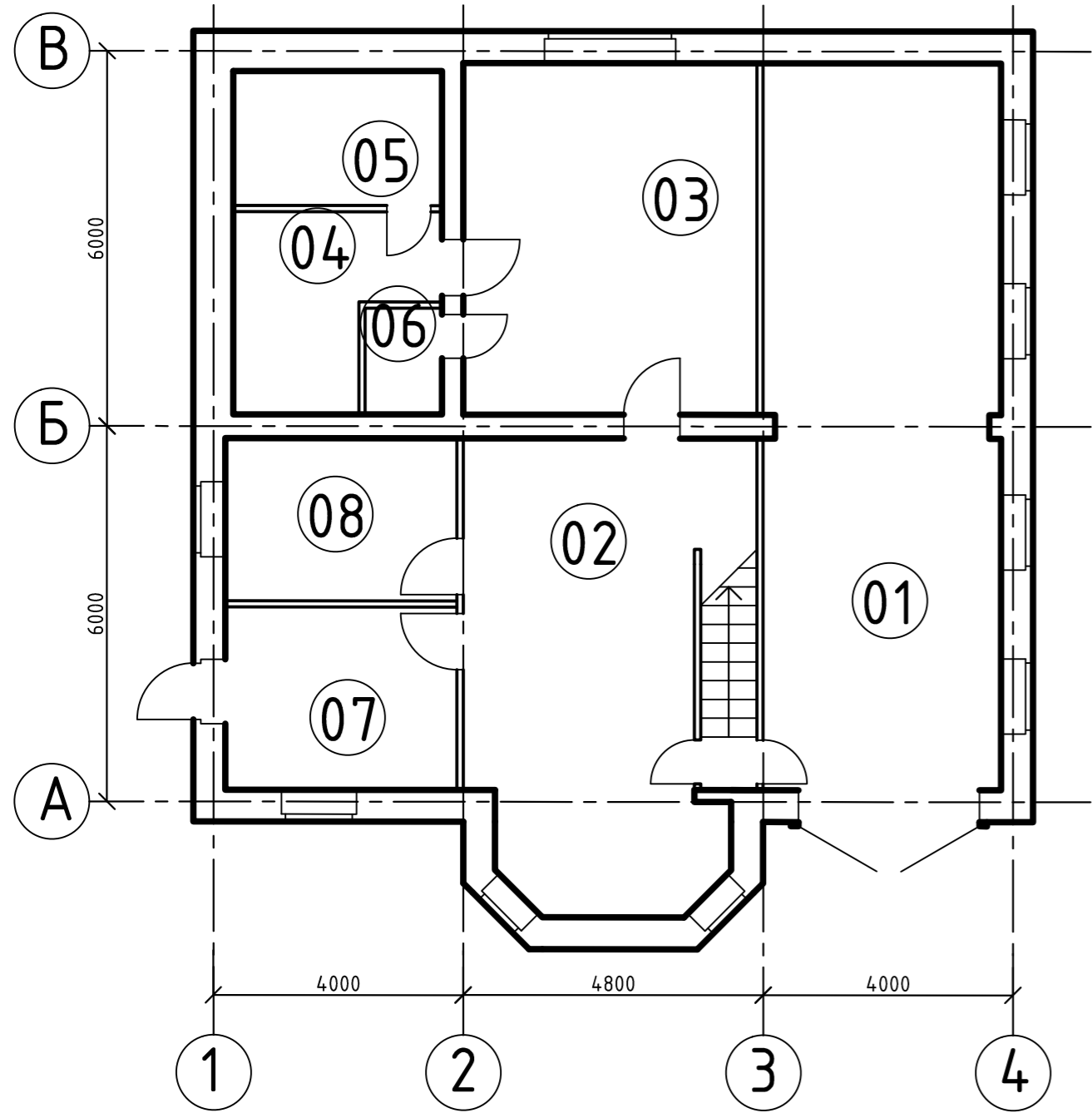
ПЛАН ЦОКОЛЬНОГО ЭТАЖА М 1:100
