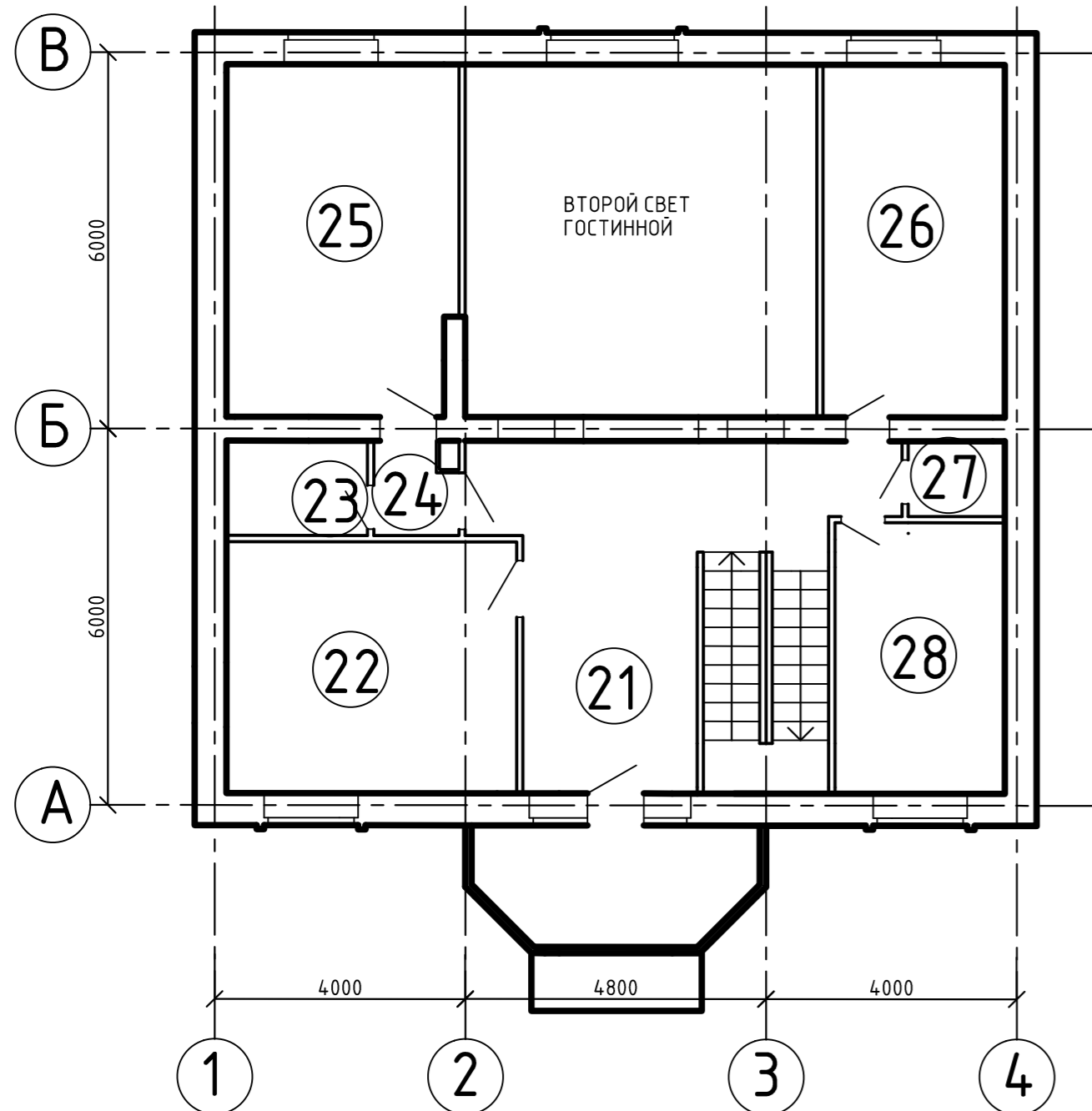
ПЛАН ВТОРОГО ЭТАЖА М 1:100
