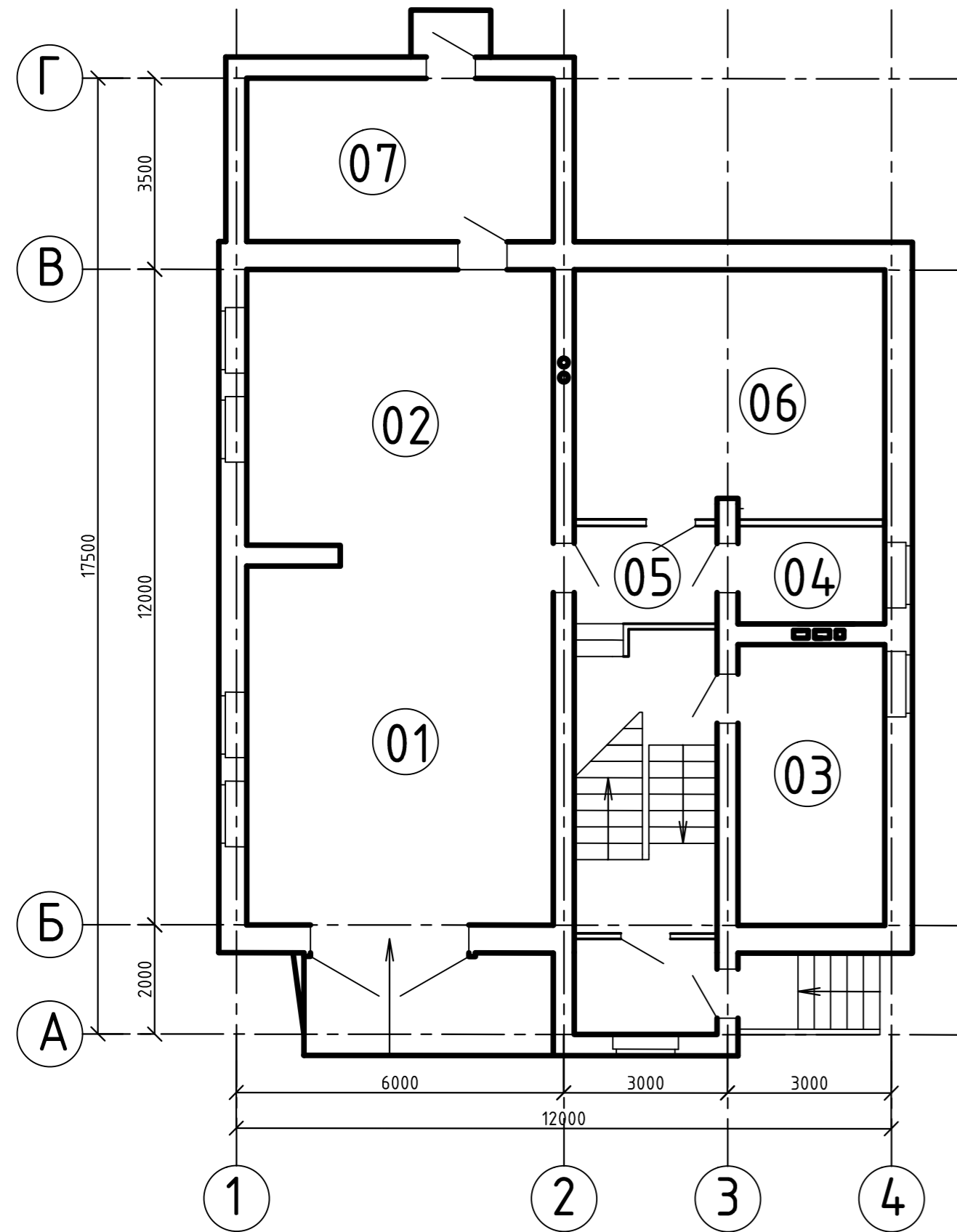
ПЛАН ЦОКОЛЬНОГО ЭТАЖА М 1:100
