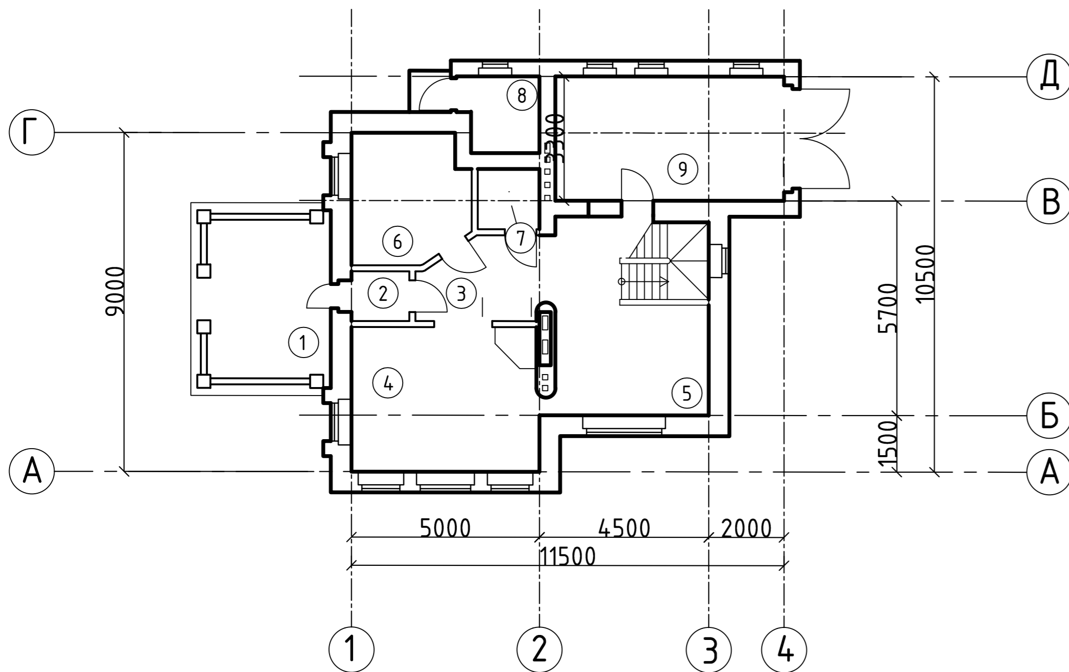
ПЛАН ВТОРОГО ЭТАЖА М 1:100
