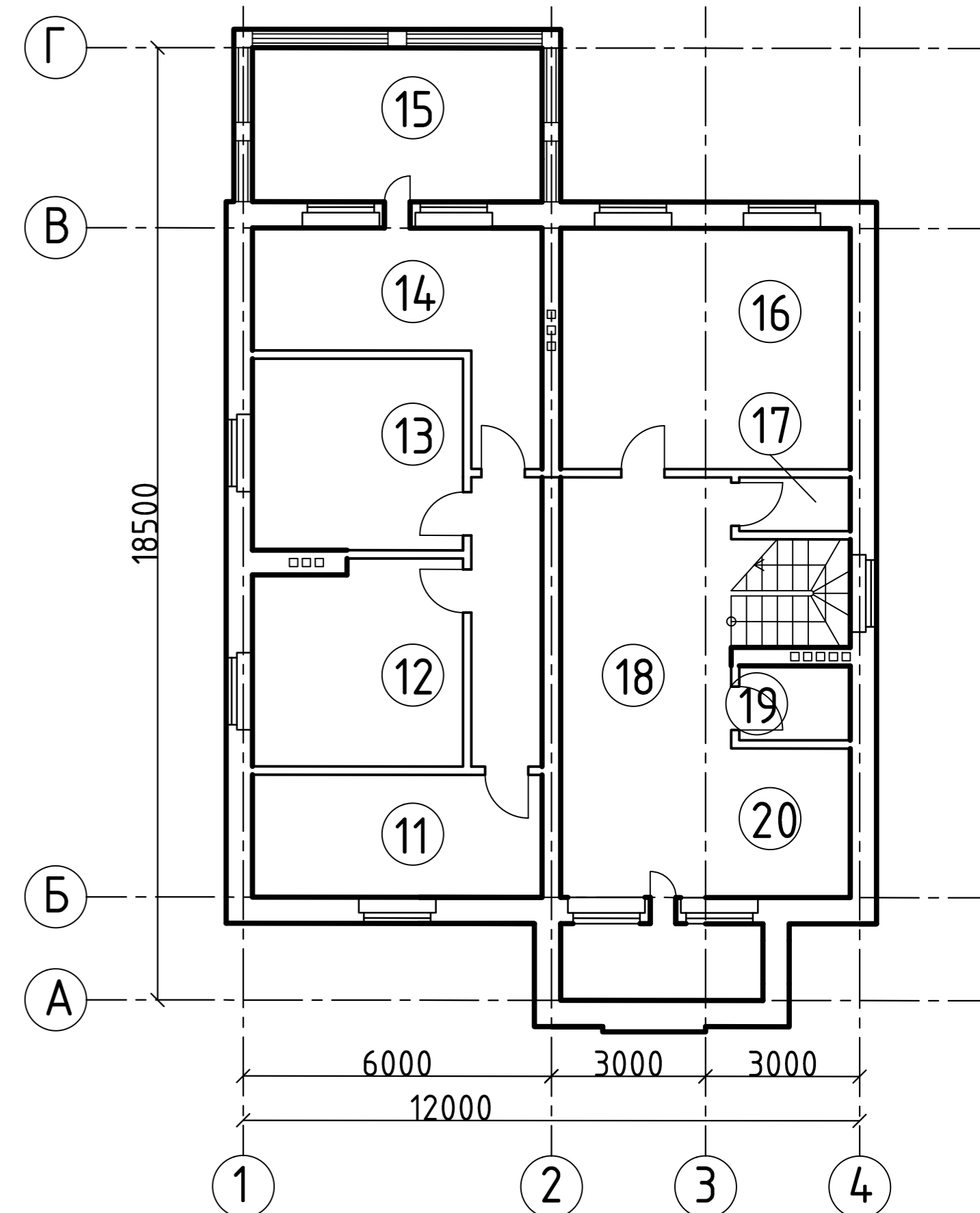
ПЛАН ВТОРОГО ЭТАЖА М 1:100
